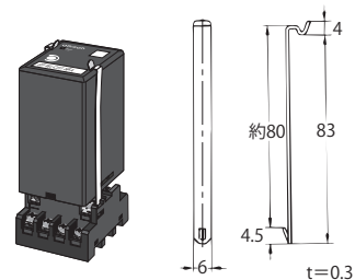
注.安裝支架PFC-N8型 (隨附於本體)
