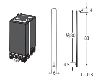
注.安裝支架PFC-N8型 (隨附於本體)
