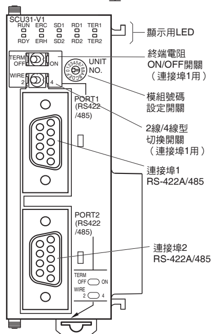
CJ1W-SCU31-V1型
