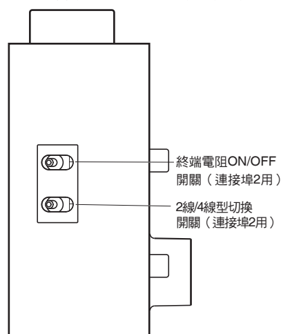
底面圖 (僅CJ1W-SCU3□ (-V1) 型)
