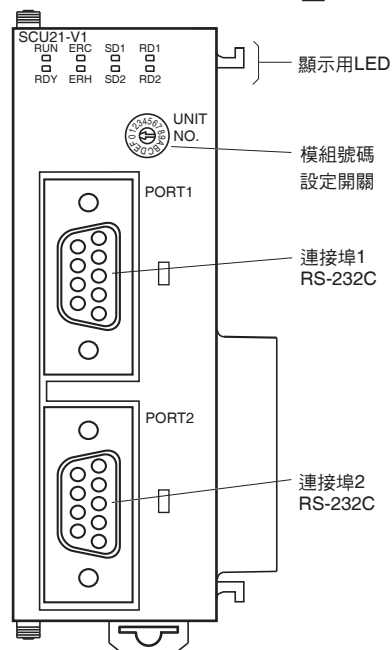
CJ1W-SCU21-V1/SCU22型
