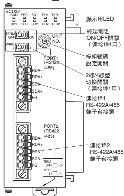
CJ1W-SCU32型
