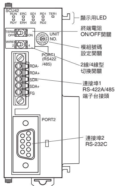
CJ1W-SCU42型
