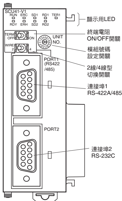
CJ1W-SCU41-V1型
