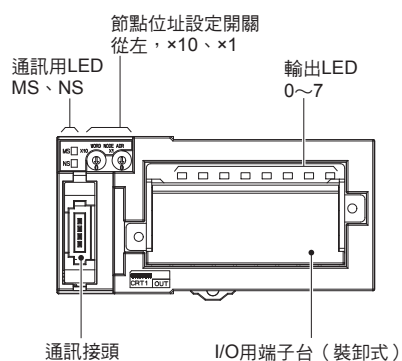
CRT1-OD08TA (-1) 型、CRT1-OD08TAH (-1) 型
