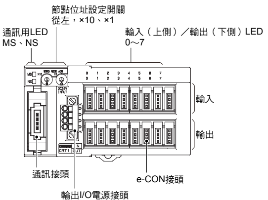
CRT1-MD16S (-1) 型、CRT1-MD16SH (-1) 型
