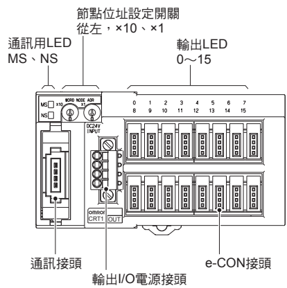
CRT1-OD16S (-1) 型、CRT1-OD16SH (-1) 型
