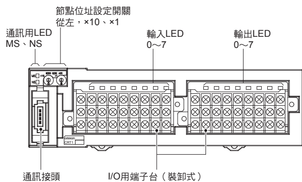
CRT1-MD16TA (-1) 型、CRT1-MD16TAH (-1) 型
