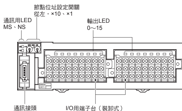
CRT1-OD16TA (-1) 型、CRT1-OD16TAH (-1) 型
