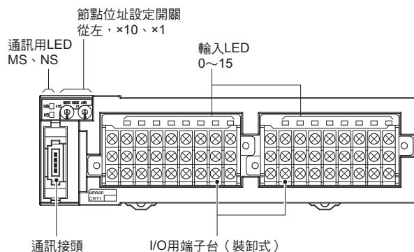
CRT1-ID16TA (-1) 型、CRT1-ID16TAH (-1) 型
