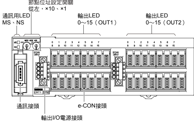
CRT1-OD32S (-1) 型、CRT1-OD32SH (-1) 型
