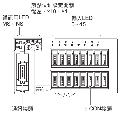
CRT1-ID16S (-1) 型、CRT1-ID16SH (-1) 型
