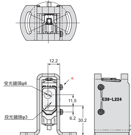
安裝感測器時的尺寸 (例：E3AS-HL500□)
