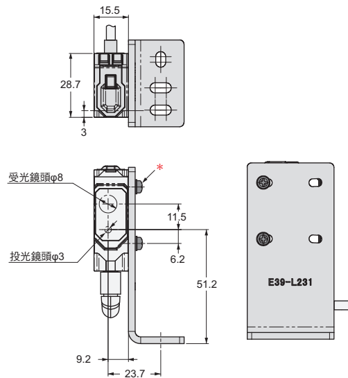
安裝感測器時的尺寸 (例：E3AS-HL500□)
