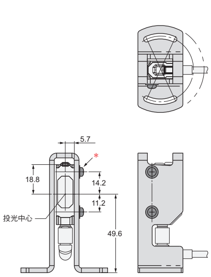
安裝感測器時的尺寸 (例：E3AS-F1500□)
