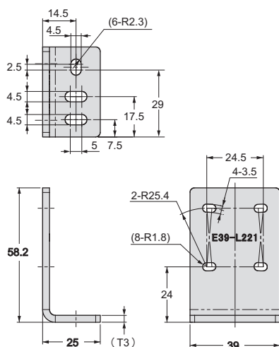
安裝感測器時的尺寸 (例：E3AS-HL500□)
