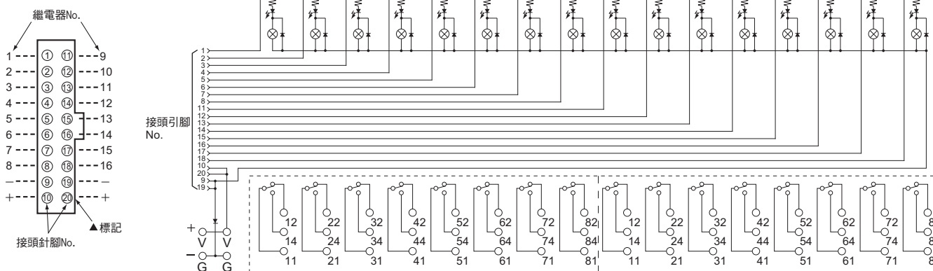
連接器引腳配置 (TOP VIEW)
