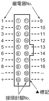
連接器引腳配置 (TOP VIEW)
