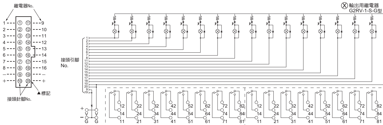
連接器引腳配置 (TOP VIEW)
