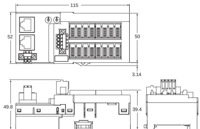
GX-OD1618/OD1628型 GX-MD1618/MD1628型
