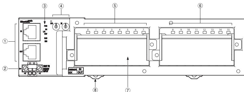
8點輸入/8點輸出端子 GX-MD1612/MD1622型
