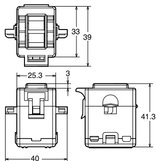
CT貫穿孔內徑尺寸
