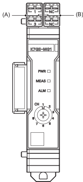
探測模組 K7GE-MG1型
