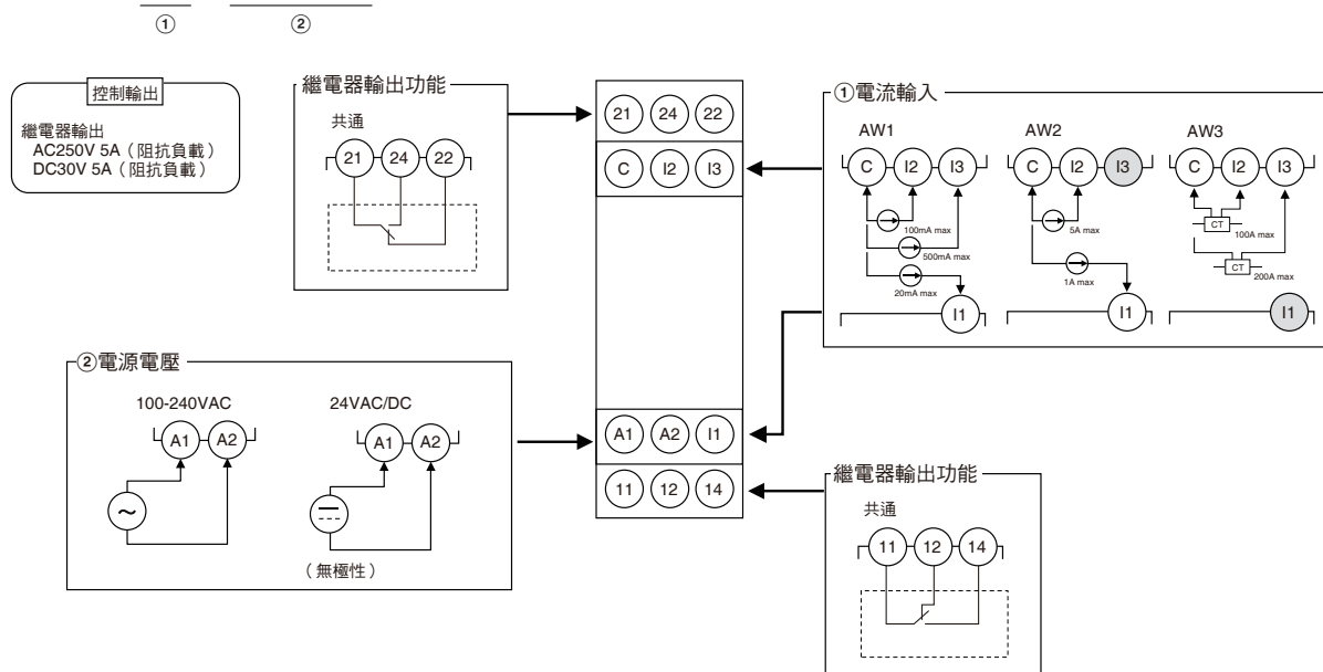
K8AK-AW1型 100-240VAC
