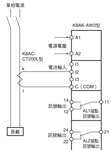
(K8AK-AW3型)
