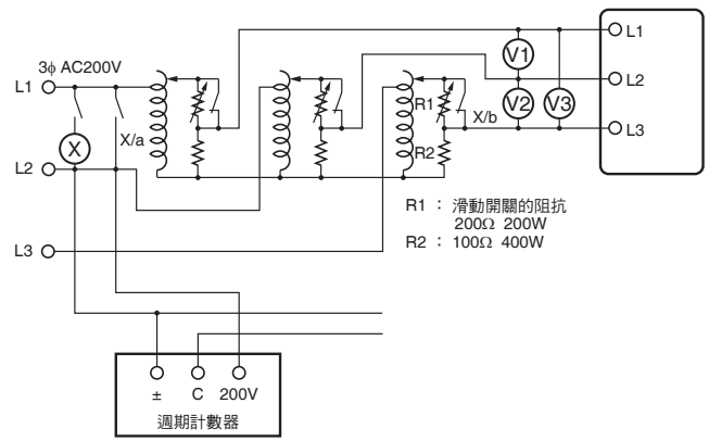
接線圖2
