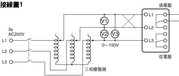
接線圖1
