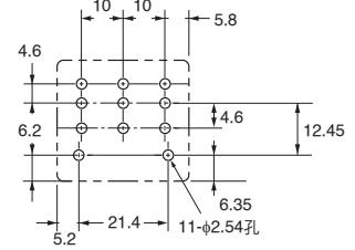
安裝孔 (底視圖)
