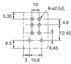
安裝孔 (底視圖)
