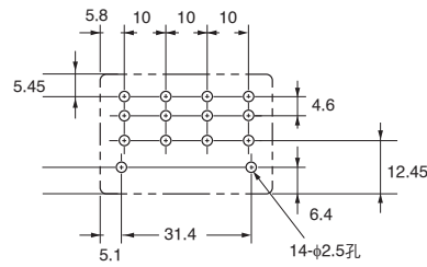
安裝孔 (底視圖)
