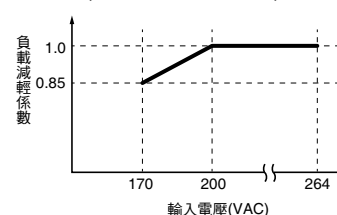
對輸入電壓之負載減輕係數
