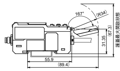
護蓋、按鈕開啟位置 (安裝 DIN 鋁軌)
