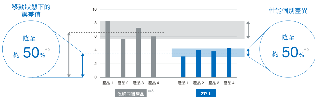
移動狀態下的測量值誤差（移動解析度） [ \mu m]
