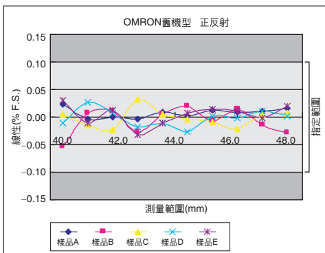
線性特性
