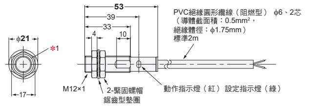
E2EF-X3D1型 E2EF-QX3D1型
