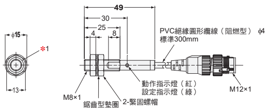
E2EF-X2D1-M1TGJ型 E2EF-QX2D1-M1TGJ型
