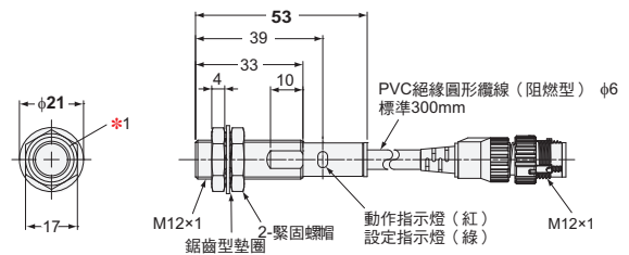
E2EF-X12D1-M1TGJ型 E2EF-QX12D1-M1TGJ型
