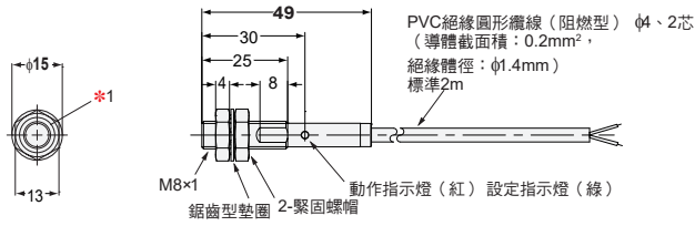
E2EF-X2D1型 E2EF-QX2D1型
