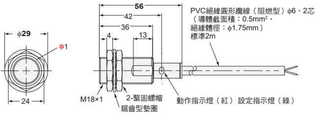
E2EF-X7D1型 E2EF-QX7D1型
