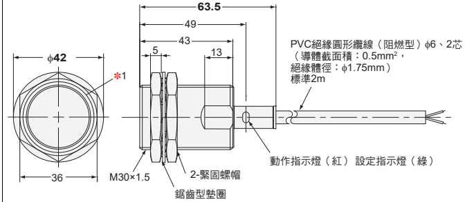
E2EF-X12D1型 E2EF-QX12D1型
