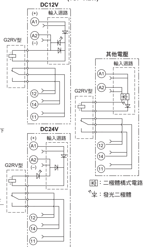
端子配置/內部接線圖 (TOP VIEW)
